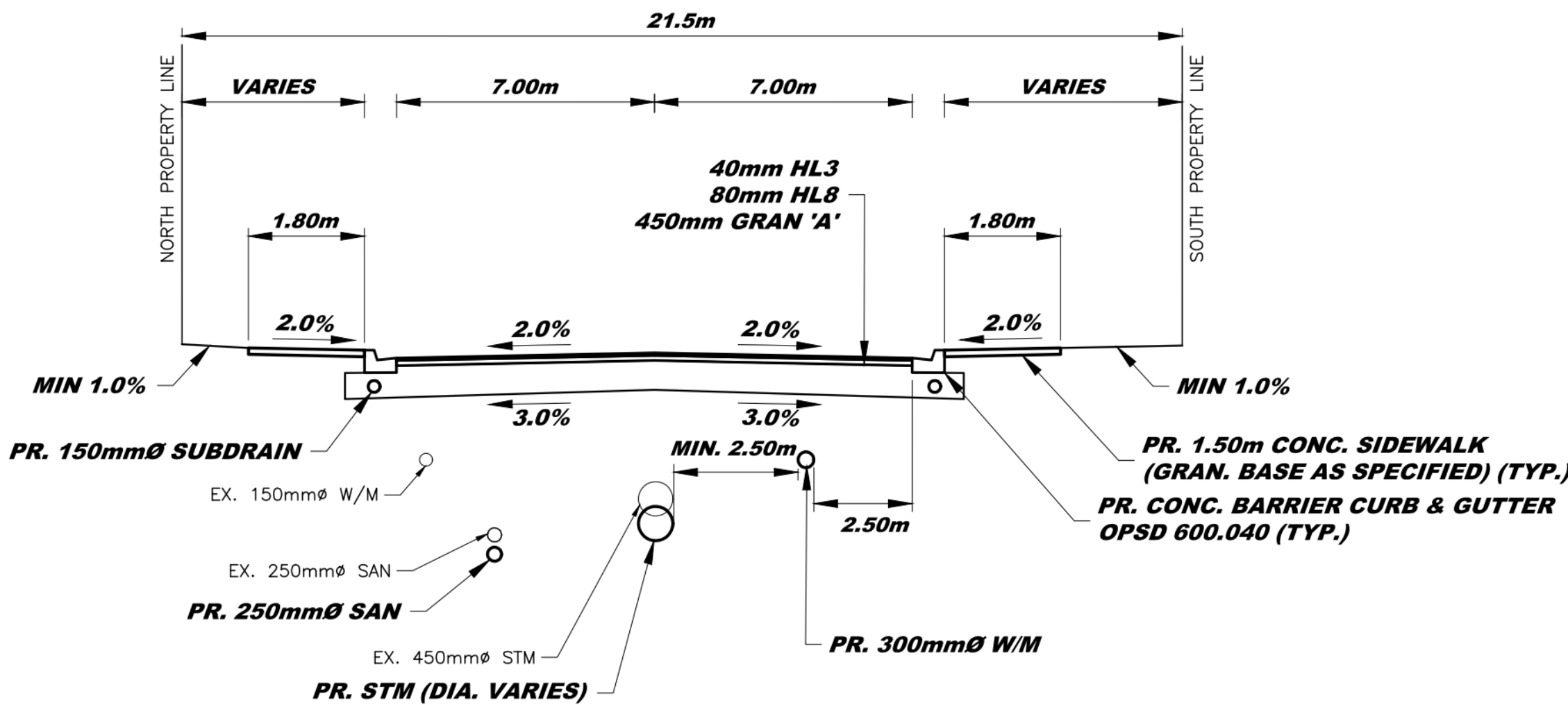
STREET A FROM STA 0+060 TO STA 0+140 N.T.S.
